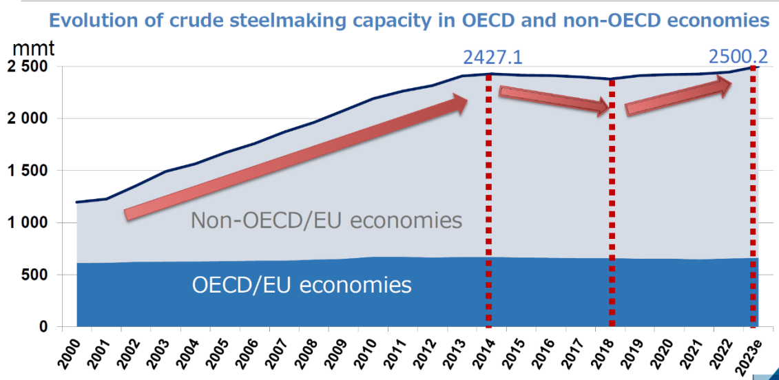
Gráfico 2. Evolución de la capacidad instalada en países OECD y No -OECD
