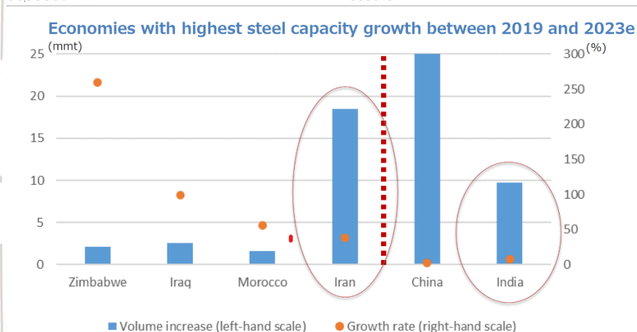
Gráfico 4. Economías con mayores crecimientos en su capacidad instalada (2019 – 2023 e)
